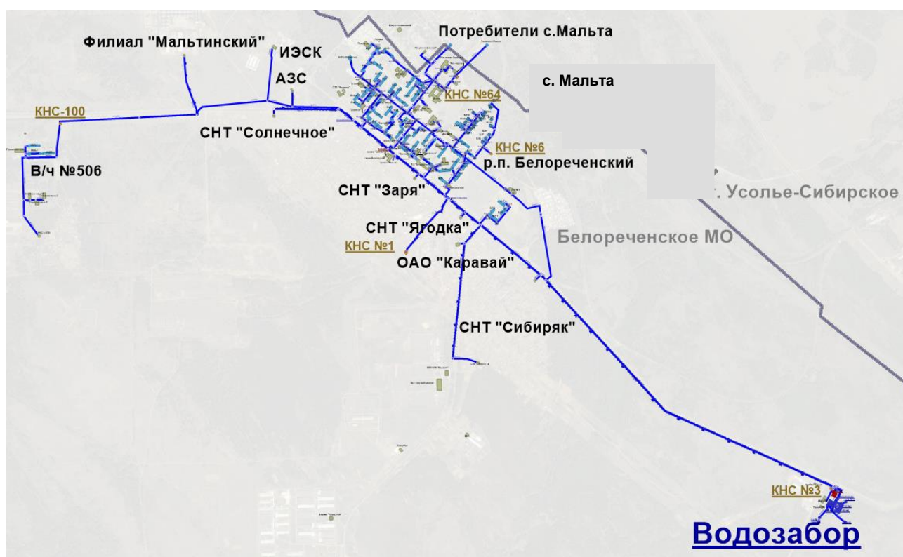
Рис. 1.1. Общая принципиальная схема централизованного водоснабжения р.п. Белореченский
