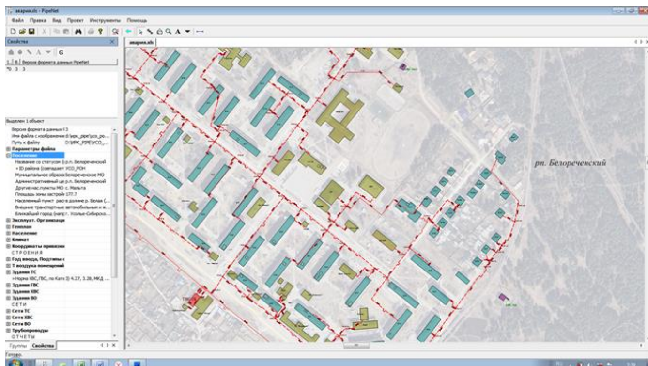
Рис. 1.1 Общий вид (фрагмент) электронной модели системы теплоснабжения р.п. Белореченский в программе PipeNet
